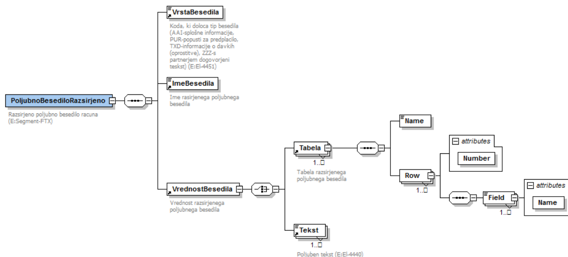
Slika 2: Vizualizacija XML sheme za element <PoljubnoBesediloRazsiruteno>
